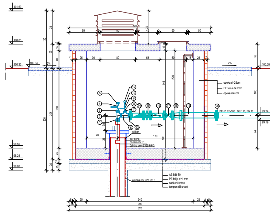
PRESEK A-A
